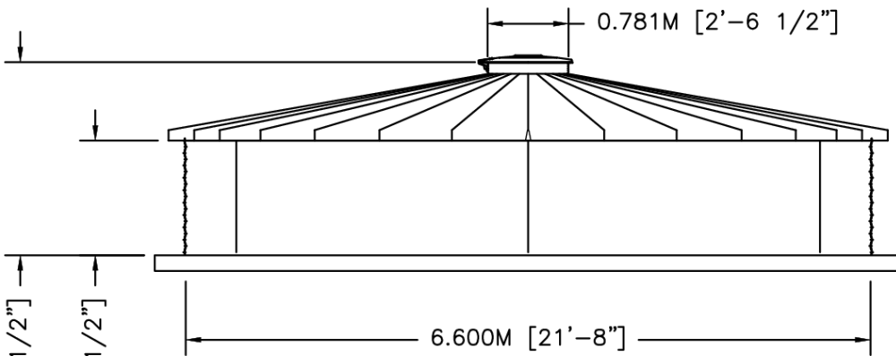
ELEVATION
